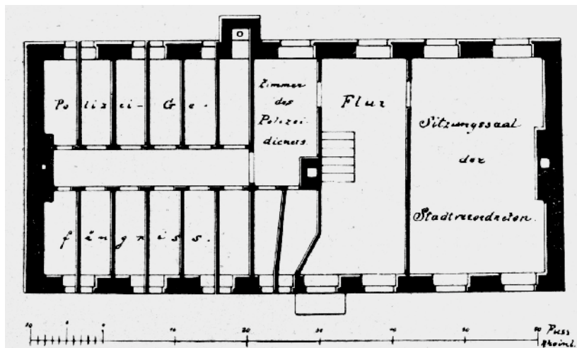
Möglicher Grundriss des zweiten Rathauses am Markt.
